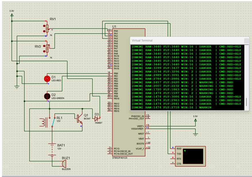
Figure 6: Kondisi DANGER - Respon Instan Lonjakan Transien Tajam dengan Penyusutan Jendela (WIN:2) dan Perintah Kombinasi Aktuator Keselamatan (CMD:RED+RLY).
