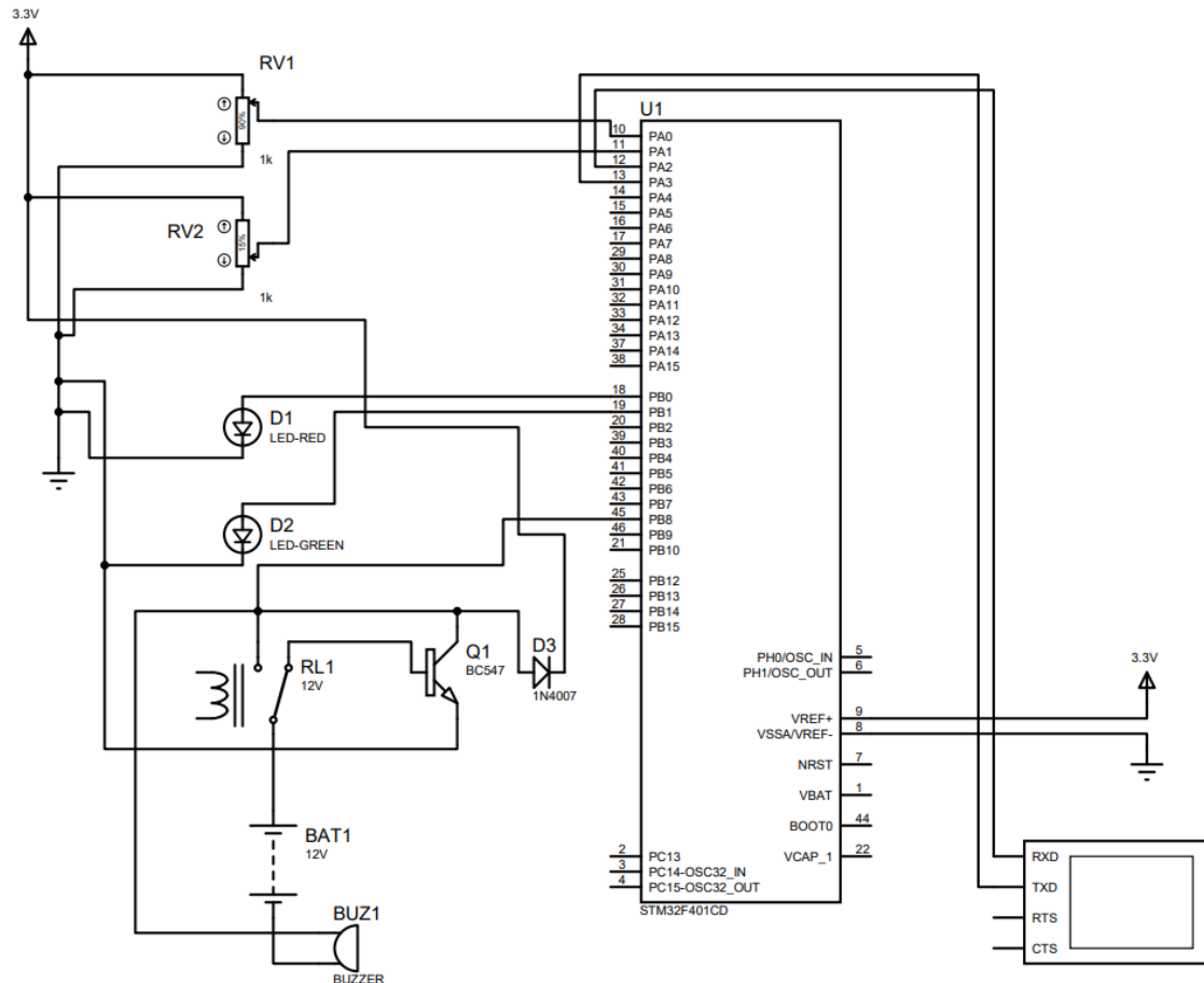
Figure 3: Skema Lengkap Rangkaian Simulasi Sistem Instrumentasi Kebakaran DMCM-WVAF pada Lembar Kerja Simulator Proteus menggunakan Target IC STM32F401CD.
